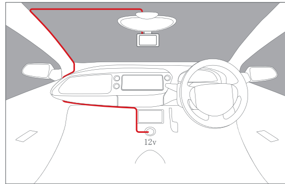
建议的摄像机电缆布线。
